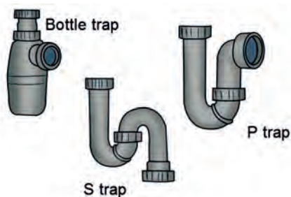
Fig. 5.17: Trap
